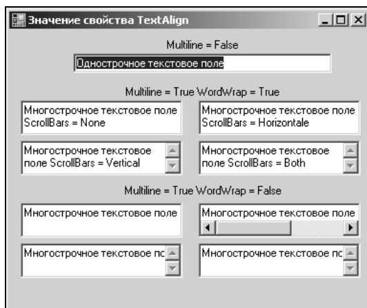
Рис. 4.2. Вид текстового поля в зависимости от значения его свойств
