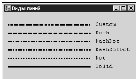
Рис. 8.1. Виды линий
