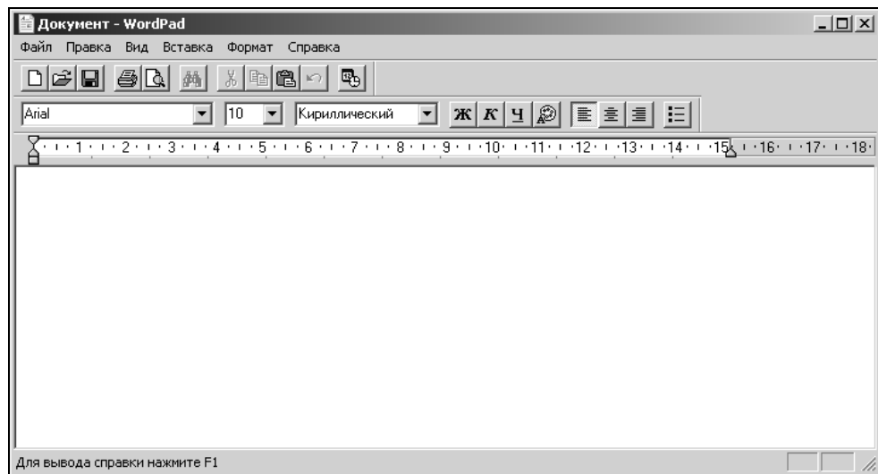
Рис. 3.9. Пример SDI-интерфейса
