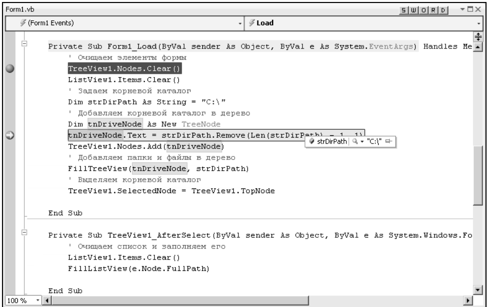
Рис. 16.3. Просмотр значения выражения в точке останова
