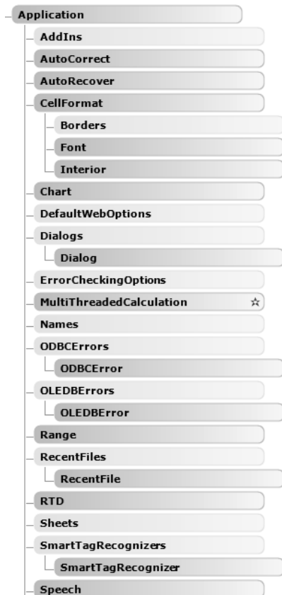
Рис. 15.3. Фрагмент объектной модели Excel
