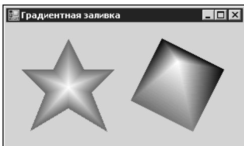
Рис. 8.19. Градиентная заливка, построенная с помощью класса PathGradientBrush
