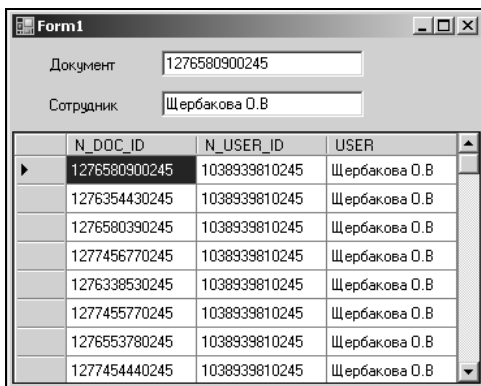
Рис. 11.10. Отображение данных с помощью свойства DataBindings
